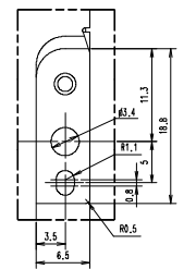
DETAIL *D*(S:3/1)
