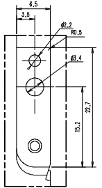
DETAIL *C*(S:3/1)
