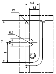
DETAIL *A*(S:3/1)
