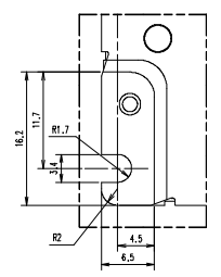
DETAIL *B*(S:3/1)
