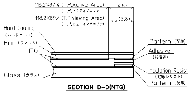
SECTION D-D(NTS)
